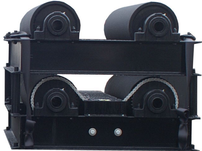
Rodillos para girar el haz con accionamiento hidráulico.
